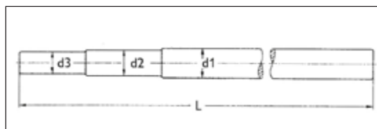
DIN 900, verchromt
